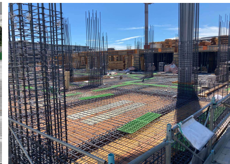
2階躯体工事
