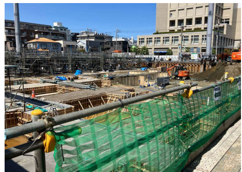
基礎工事
