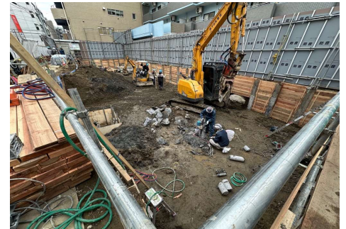
山留工事
