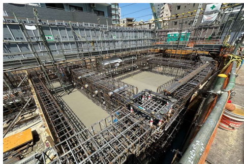
基礎工事
