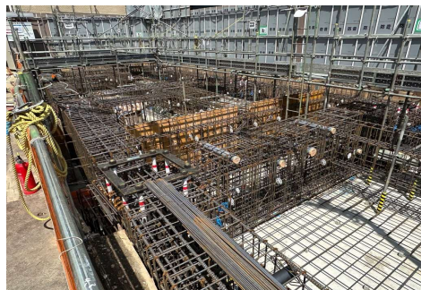
基礎工事
