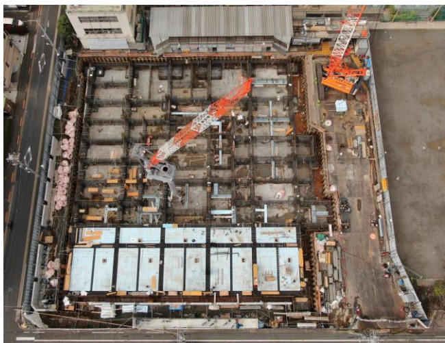
1階躯体工事
