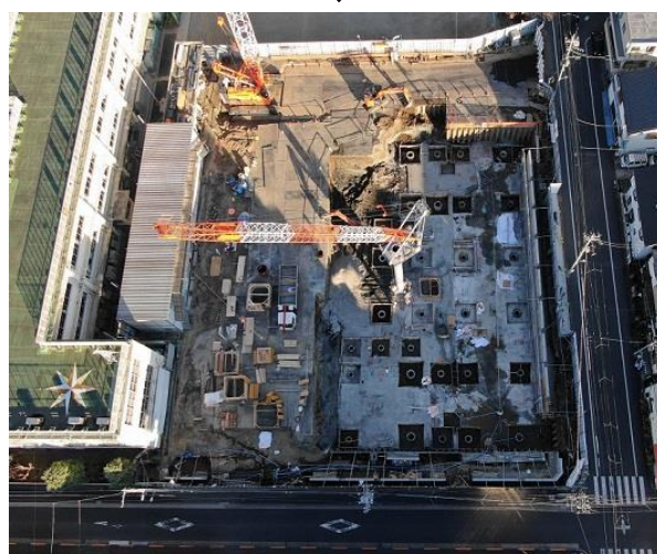
基礎工事
