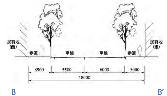
道路断面図（B-B'断面）
